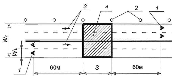
б) четырехполосная дорога с двусторонним движением и односторонним расположением ОП
