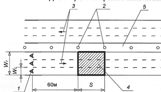
г) шестиполосная дорога с разделительной полосой и центральным расположением ОП
