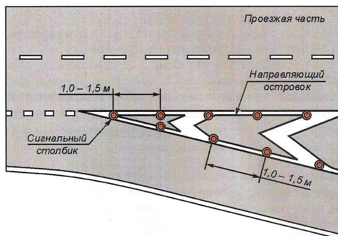
Рисунок 9 — Установка столбиков на направляющих островках
