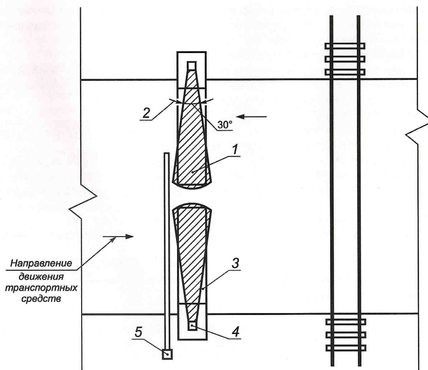
1 — диаграмма направленности; 2 — ширина диаграммы направленности; 3 — крышка ЗД; 4 — КЗК; 5 — шламбаум
