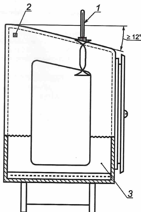
1 — термометр; 2 — клапан сброса давления; 3 — поддон наполненный водой
