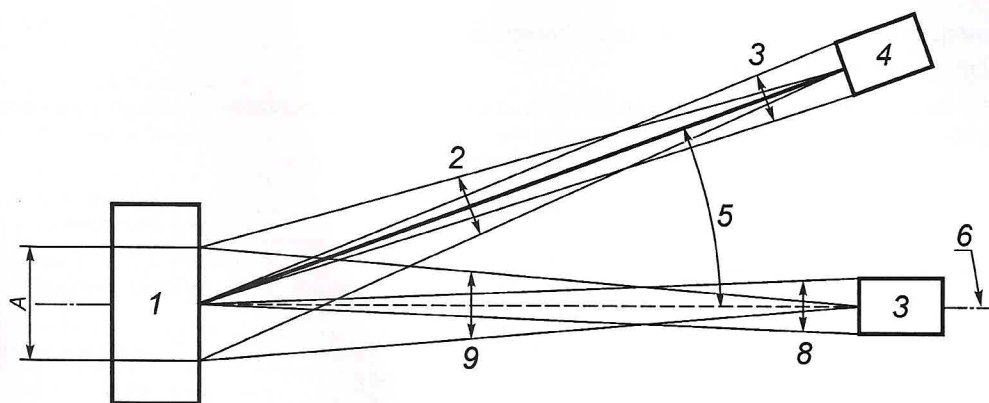
A — диаметр области измерения; 1 — испытательный модуль; 2 — не более 3^\circ ; 3 — не более 2^\circ ; 4 — солнечный имитатор; 5 — (10 \pm 0,1)^\circ и (5 \pm 0,1)^\circ для класса L3(*); 6 — ось отсчета; 7 — яркомер; 8 — не более 5^\circ ; 9 — не более 3^\circ
