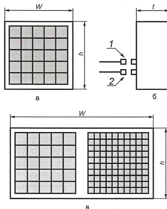
а, в — виды спереди; б — вид сбоку; 1 — ввод питания; 2 — ввод управления; w — ширина; h — высота; t — толщина. Закрашенные прямоугольники являются эквивалентными областями элементов и образуют область проверки светотехнических характеристик
