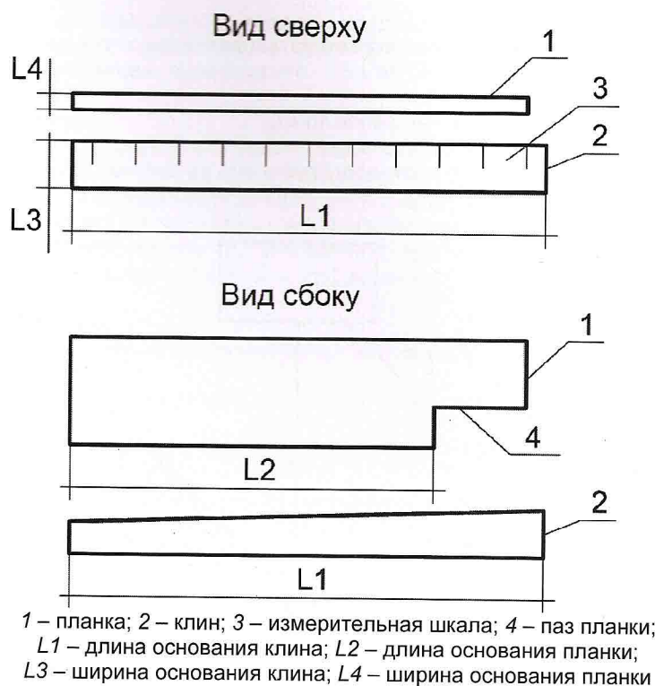
Рисунок 9 – Схема высотомера для определения высоты выступания горизонтальной дорожной разметки над поверхностью, на которую она нанесена
