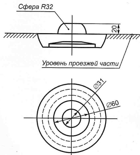
Рисунок Б.4 — Световозвращатель типа КД4
