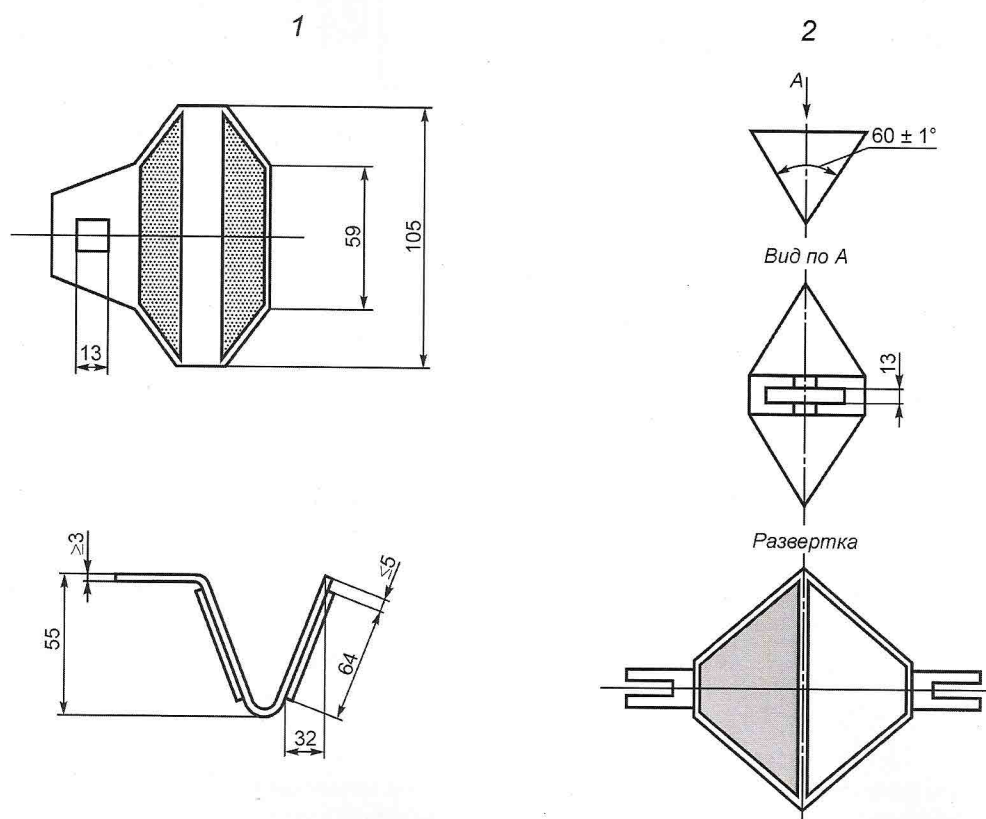
Рисунок Б.4 — Световозвращатель типа КД4
