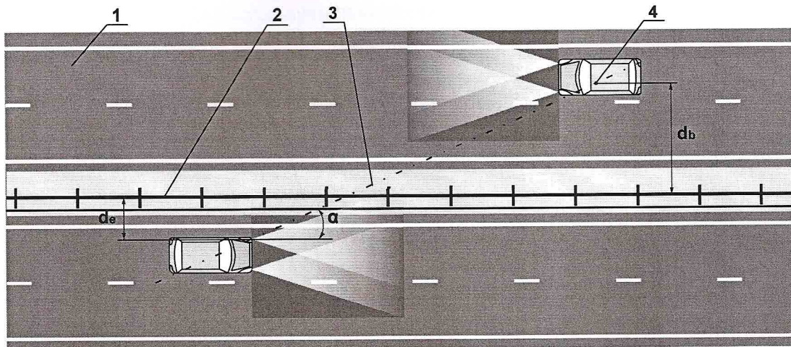
1 – проезжая часть; 2 – ось экрана; 3 – луч света; 4 – положение глаз водителя; d_e – расстояние от глаз водителя до противоослепляющего экрана; d_b – расстояние от фары транспортного средства, являющегося источником луча падающего света, до противоослепляющего экрана Рисунок Б.2 – Схема расположение транспортных средств в горизонтальной плоскости
